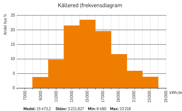
Figur 9. Uppmätt total energianvändning, summa energi för byggnadsuppvärmning, varmvatten och hushållsel för 51 direktelvärmda friliggande 1½-planshus i Källered byggda 1973. 1992/1993 uppgick medelvärdet till 18 900 kWh/år. Sedan dess har ett okänt antal energisparåtgärder utförts. Mätvärdena avser 2012.
