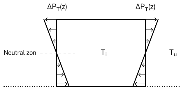
Figur 2. Tryckskillnader över klimatskärmen av olika temperatur inne och ute.
