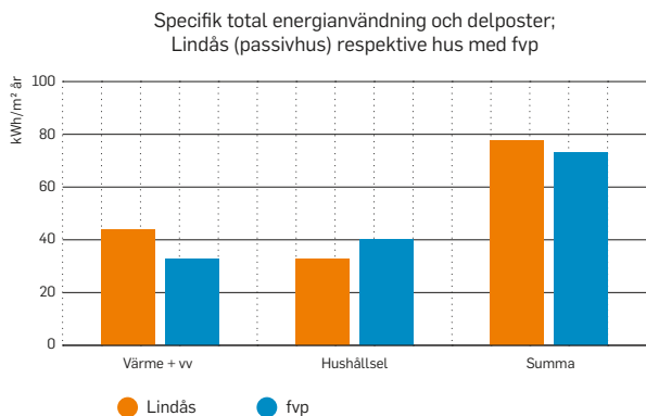
Figur 8. Välbyggda serieproducerade småhus med frånluftsvärme-pump är bättre än passivhusområdet Lindås Park.
