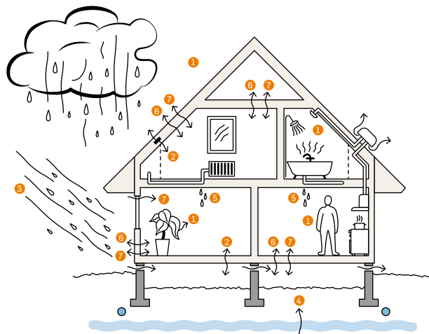
Figur 3. Fuktkällor och fukttransport sätt.
