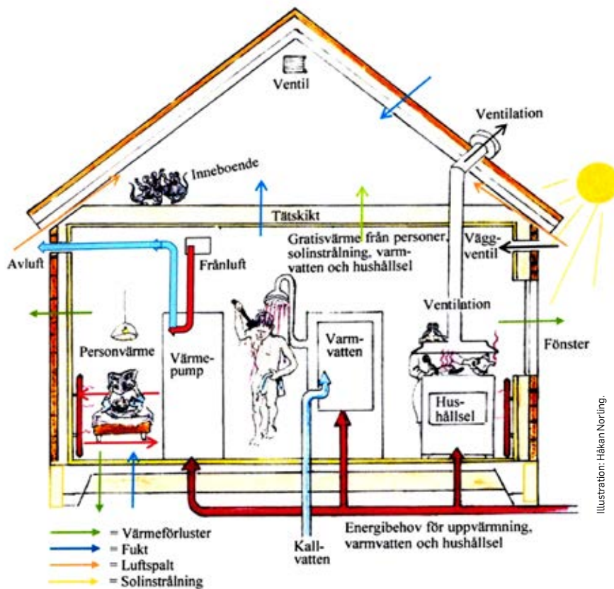
Figur 1. Vanligt energisystem i nya småhus. Schematisk beskrivning av byggteknik, värme, ventilation och återvinning.
