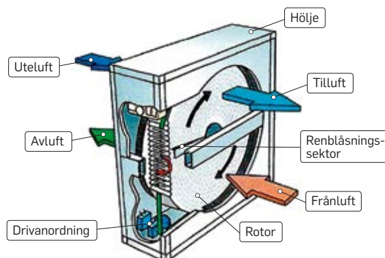
Figur 5. Roterande värmeväxlare. Energi & Miljö 1–2, 2020, Stockholm.
